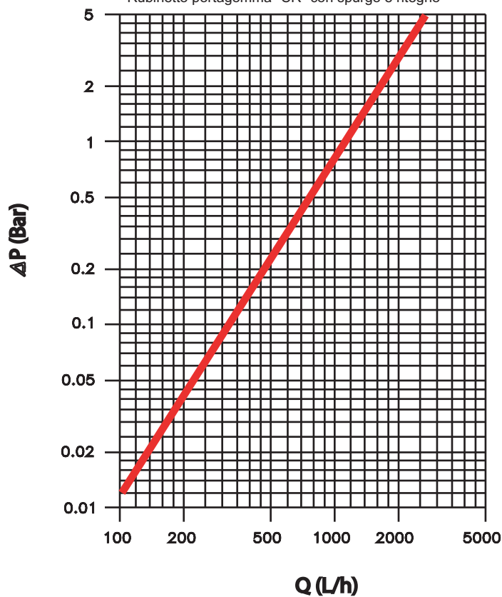
Art. 201D---S--E Rubinetto portagomma "CR" con spurgo e ritegno
